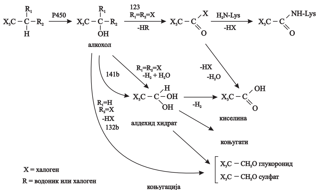
Слика 5. Метаболички путеви деградације неких фреона.
